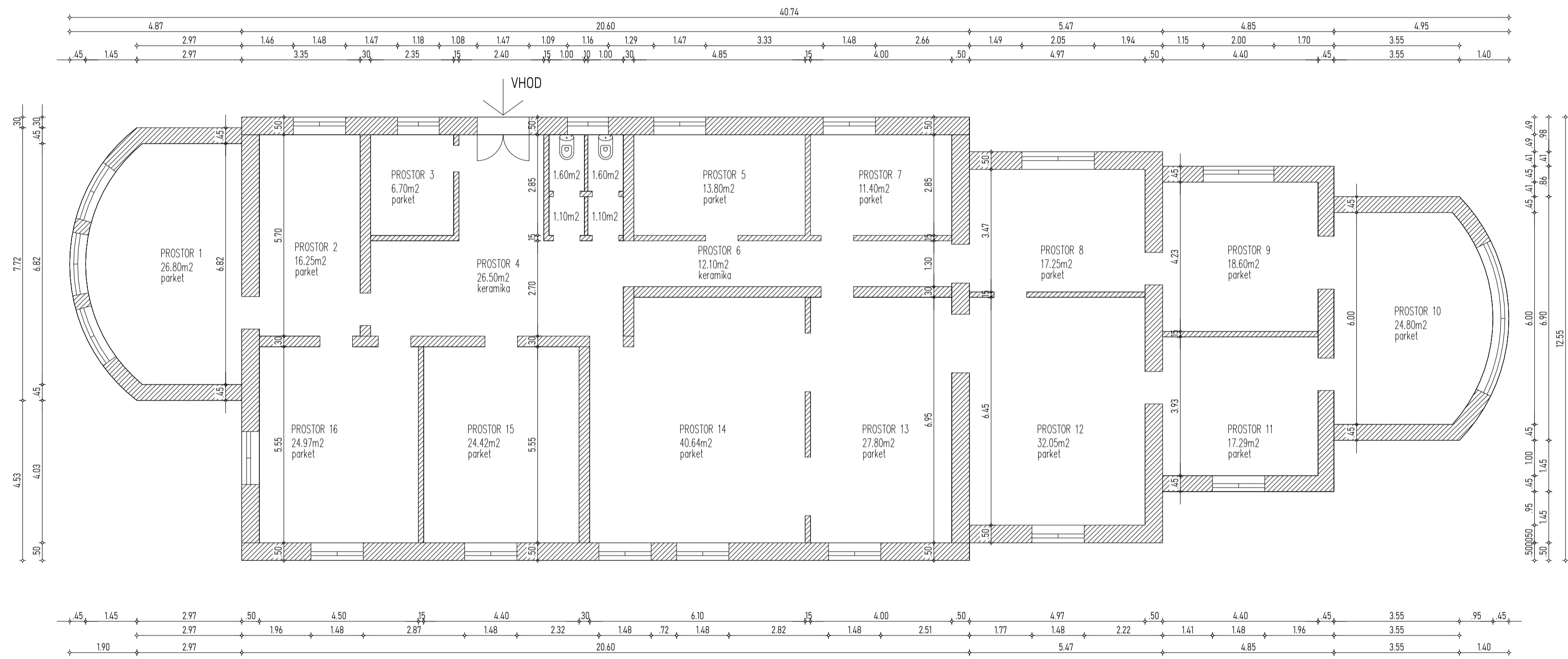
0 1m 5m TLORIS PRITLIČJA
